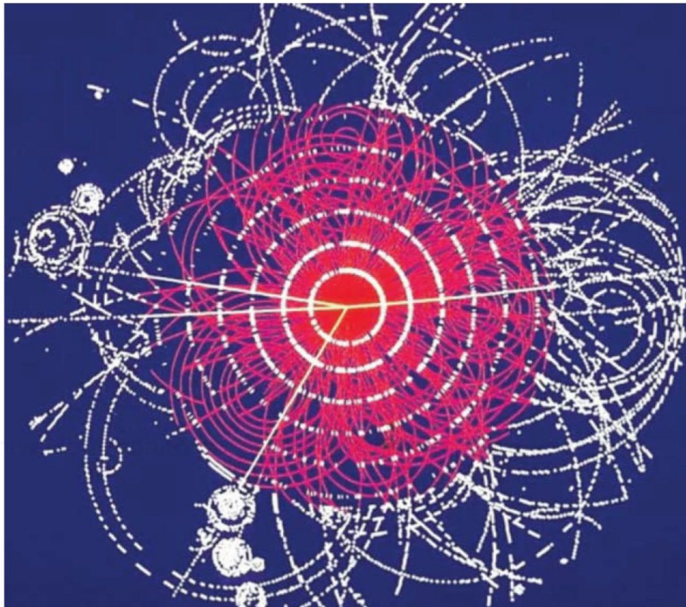
↑ Representación del modelo matemático de la Partícula de Dios o Bosón de Higgs, descubierta por Peter Higgs.
