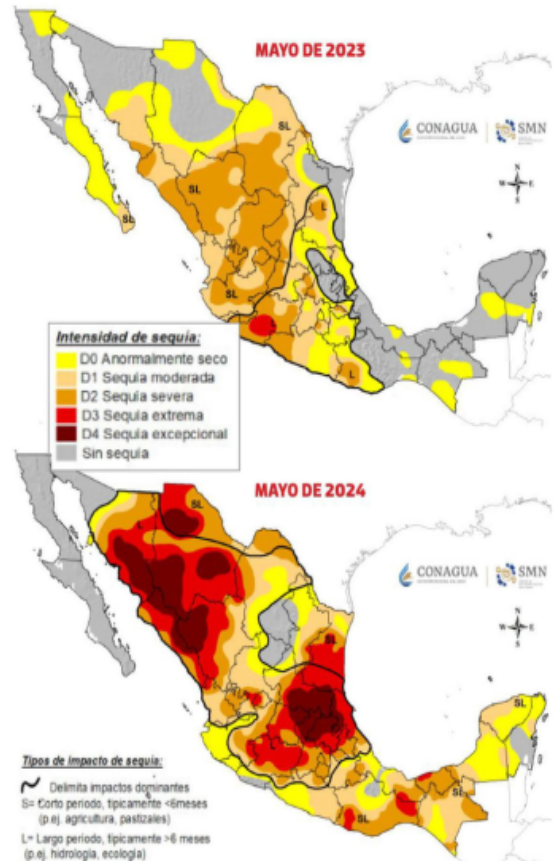
Gráficos del monitoreo de sequías en México, ambas para mayo. Arriba 2023 y abajo 2024, esta última imagen con la proliferación de las llamadas "sequías excepcionales"
