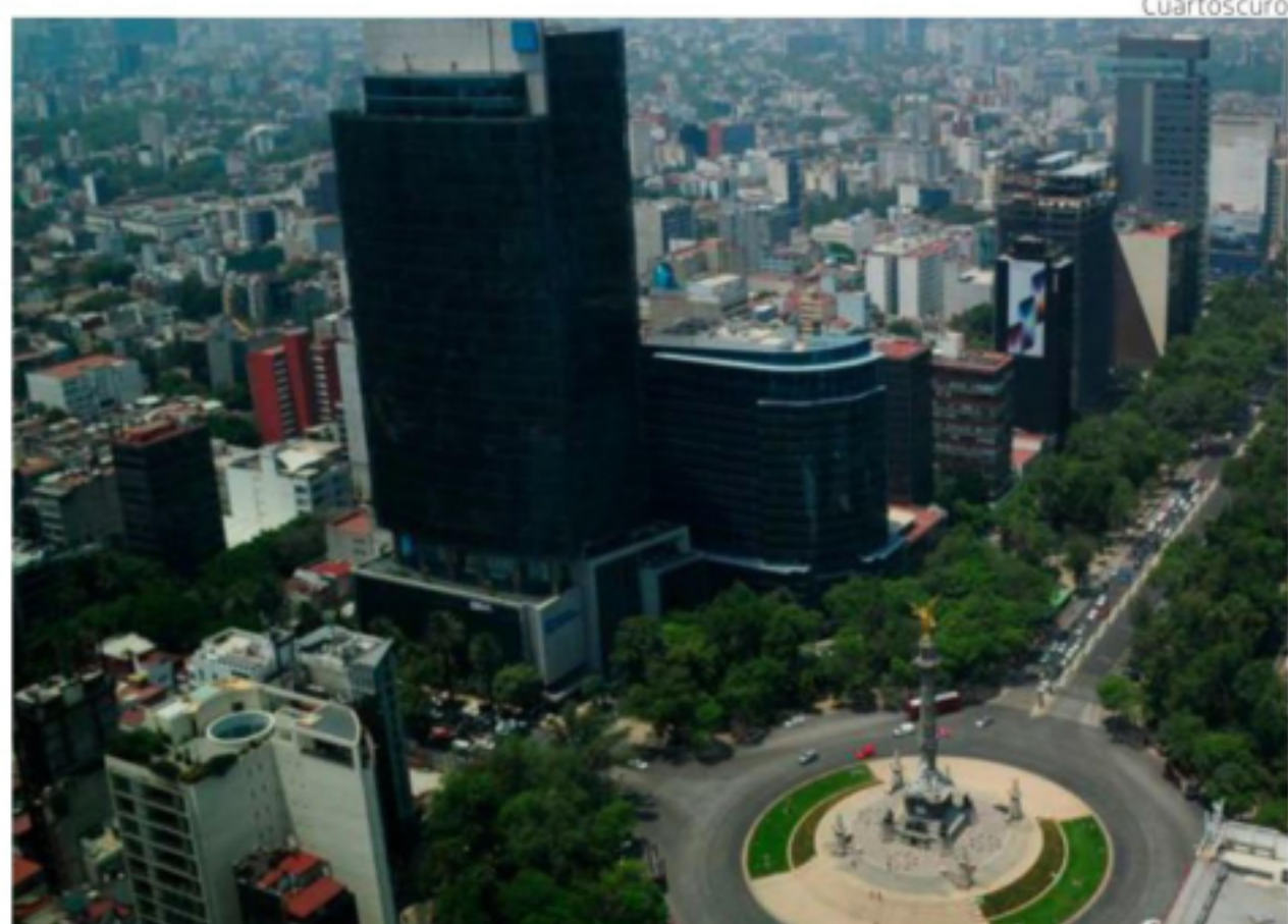
El Valle de México presentó altas concentraciones de ozono.
