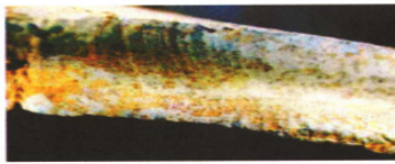
Marcas de fatiga de la grieta a lo largo de la superficie de la fractura en el alma de la viga T-6.
